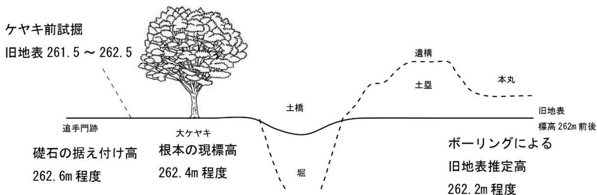
第 27 図 想定される築城以前のあり方
