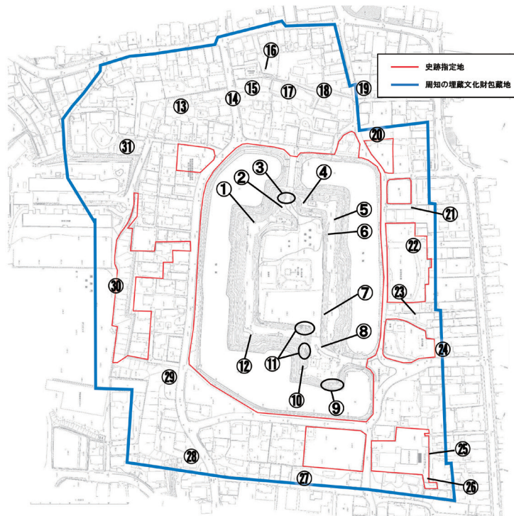
第32図 棚倉城跡現況調査の位置図
