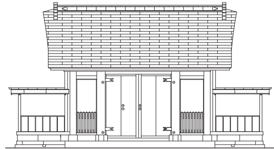
第31図 長久寺山門 立面図
