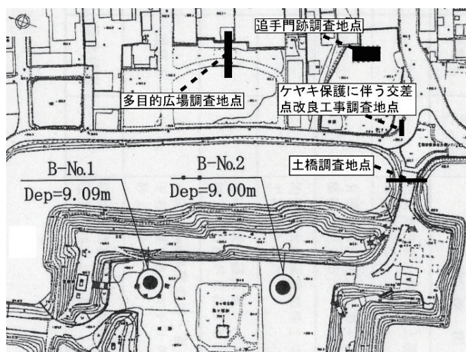
第 25 図 ボーリング調査地点
