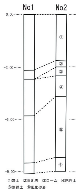
第 26 図 ボーリング調査土層模式図
