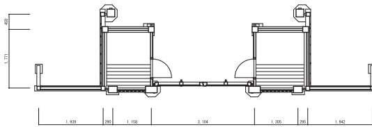
第30図 長久寺山門 平面図
