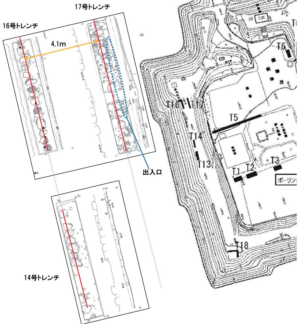
第 24 図 多門櫓礎石検出状況
