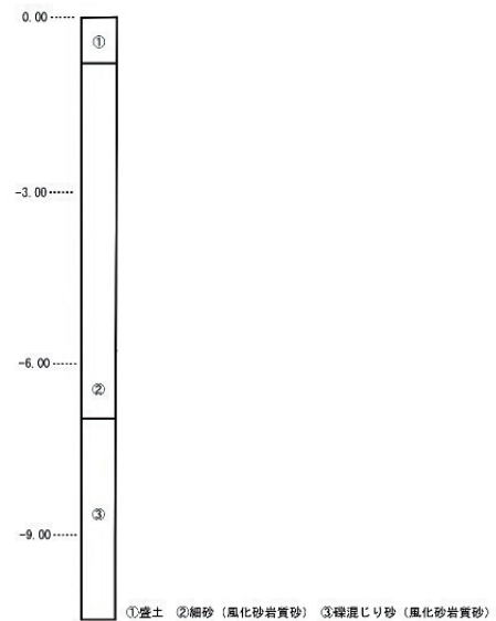
第 29 図 石垣付近ボーリング調査土層模式図
