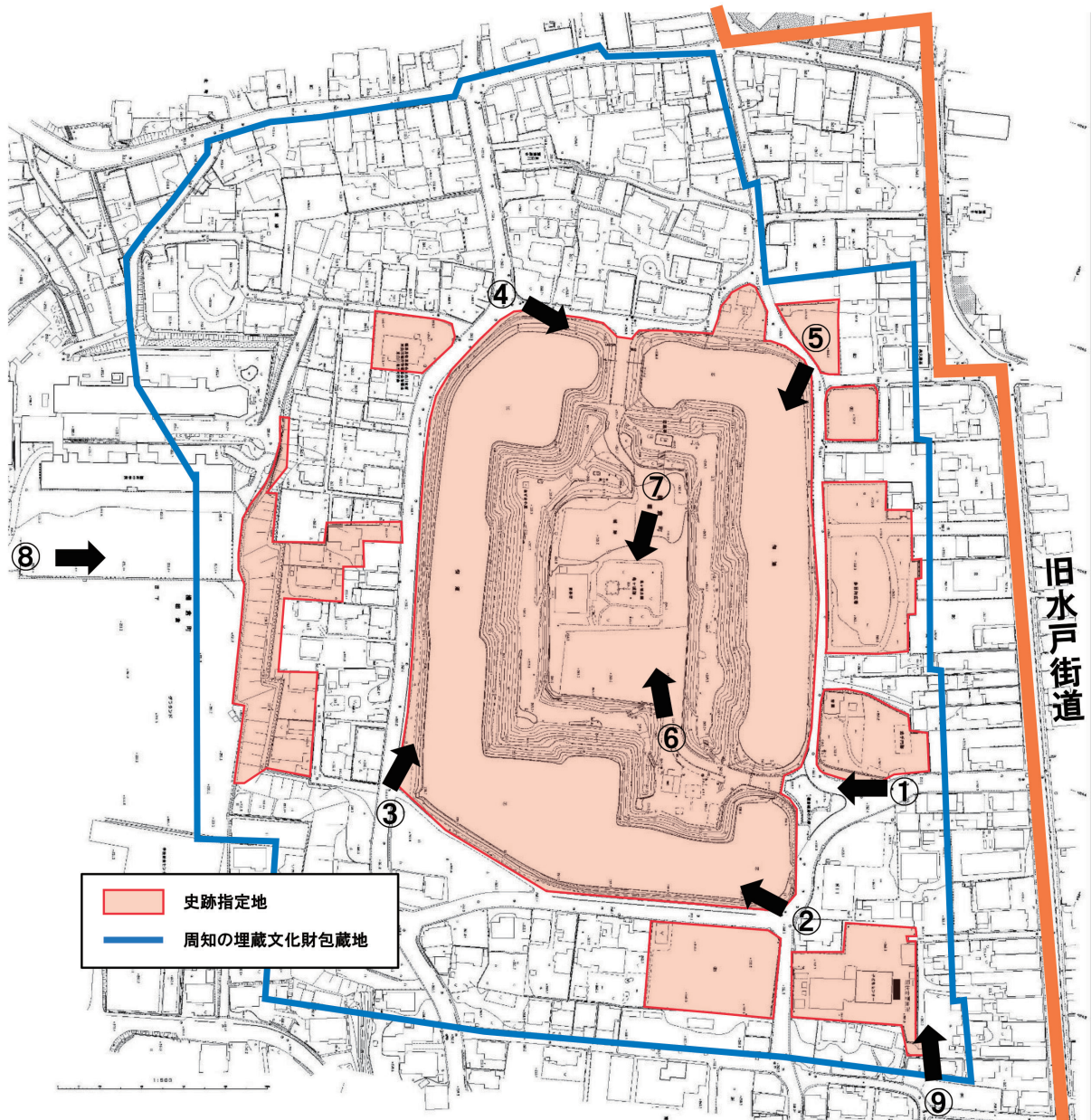
第 39 図 史跡地外部からの景観写真撮影位置図
